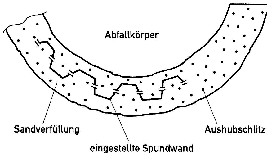
Bild 4-3.1: Schlitzaushub im Abfallkörper mit eingestellter Spundwand
